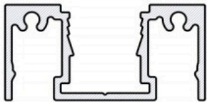
Dolo 45.01
