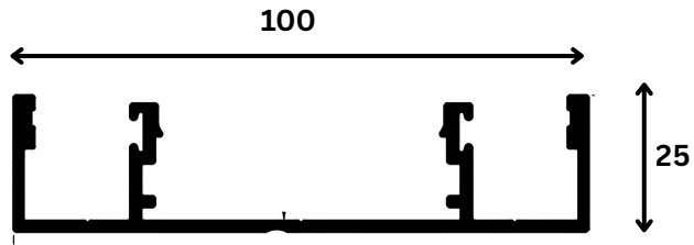
DOLO DGU 100.01
