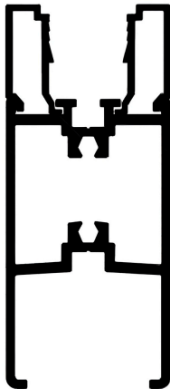
DOLO 36.02
