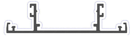
DOLO DGU 100.02
