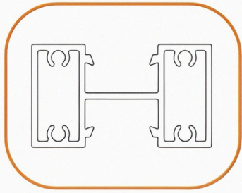
DOLO 45 H
